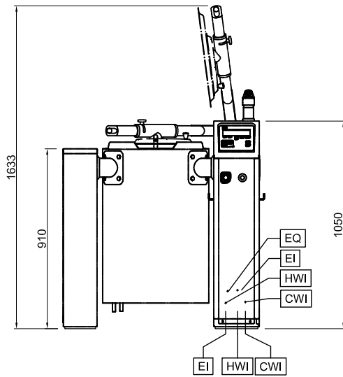
Front aanzicht
